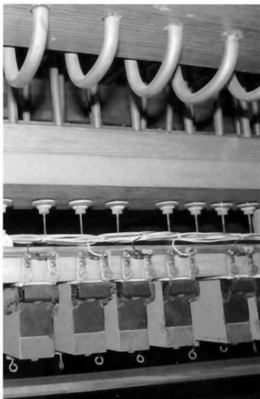
Les électro-aimants de 1928 activant les soupapes pneumatiques. Le câblage est récent. (Photo François Comment)
